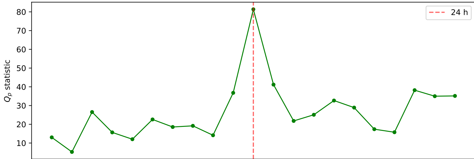
Chi-Square Periodogram
